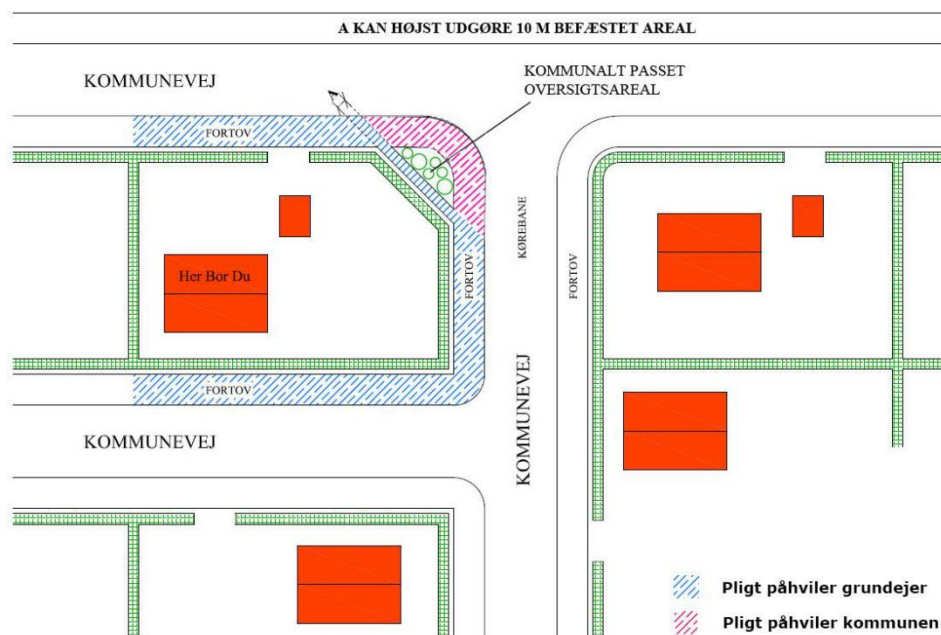
Figur 12-2 Hjørnegrund - som figur1 - hvor pligten kan pålægges grundejeren på alle sider. Her kan grundejeren dog ikke pålægges pligten rundt om oversigtsarealet, da det ikke er nærmest beliggende ejendommen.
