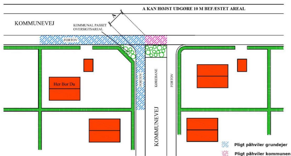
Figur 12-5 Hjørnegrund med grænser til 2 kommuneveje, hvor sidevejen er lukket fx med beplantning eller skilt. Fortovet går forbi lukningen, og pligten for fortovet forbi denne kan ikke pålægges grundejeren.
